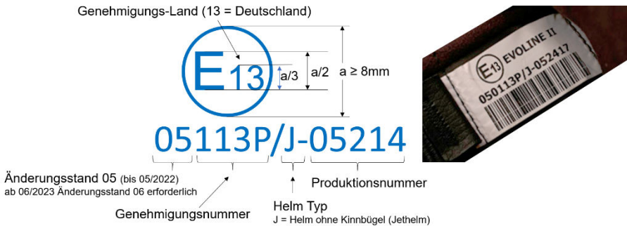
Abb. 3: Beispiel Prüfzeichen Motorradhelm
